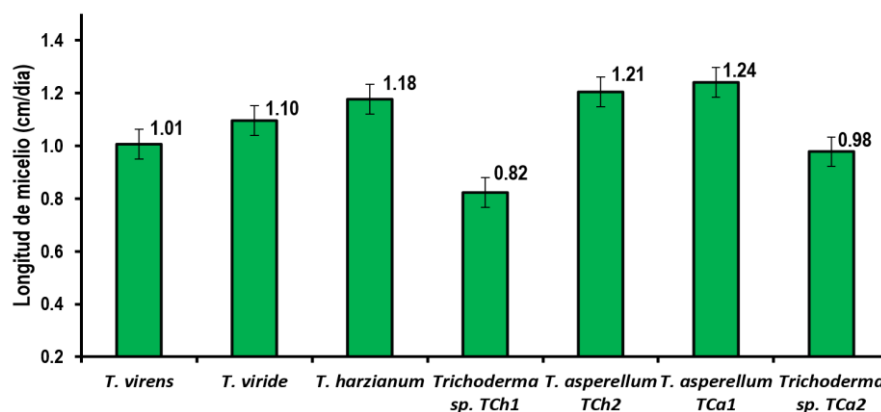
Figura 3. Tasa de crecimiento micelial de aislados de Trichoderma en medio PDA a 25 °C.
