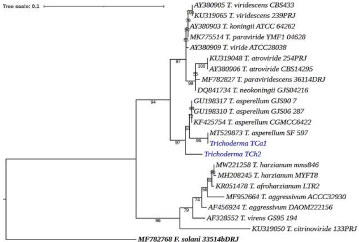
Figura 2. Árbol filogenético construido por el método de máxima verosimilitud, a partir de las secuencias nucleotídicas de ITS del GenBank y nuestros aislados (en azul), en programa IQ-TREE v. 2 y editado con ITOL, Fusarium solani es grupo externo.
