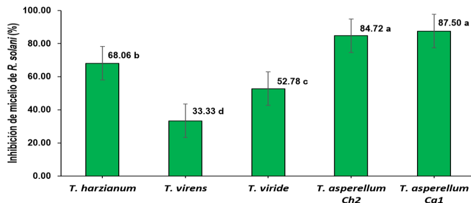
Figura 4. Inhibición del crecimiento micelial de R. solani por aislados de Trichoderma mediante el método de placas precolonizadas a los 7 días.
