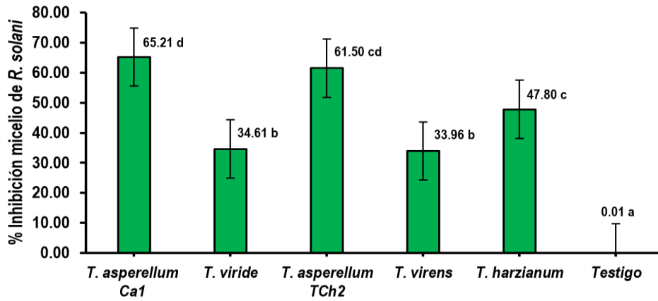
Figura 5. Inhibición del crecimiento micelial de R. solani mediante filtrados de cultivo de Trichoderma spp.
