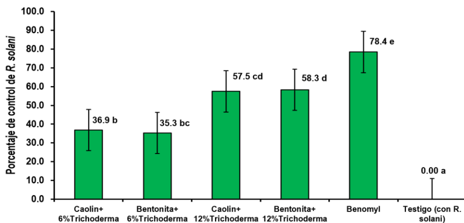
Figura 7. Porcentaje de control (eficacia) de R. solani en algodón con formulados de T. asperellum TCAL.
