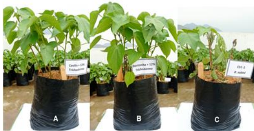
Figura 6. Crecimiento de algodón tratado con formulado polvo humectable de T. asperellum . A: Formulado en caolín + 12 % de conidias, B: bentonita + 12 % conidias, C: testigo.
